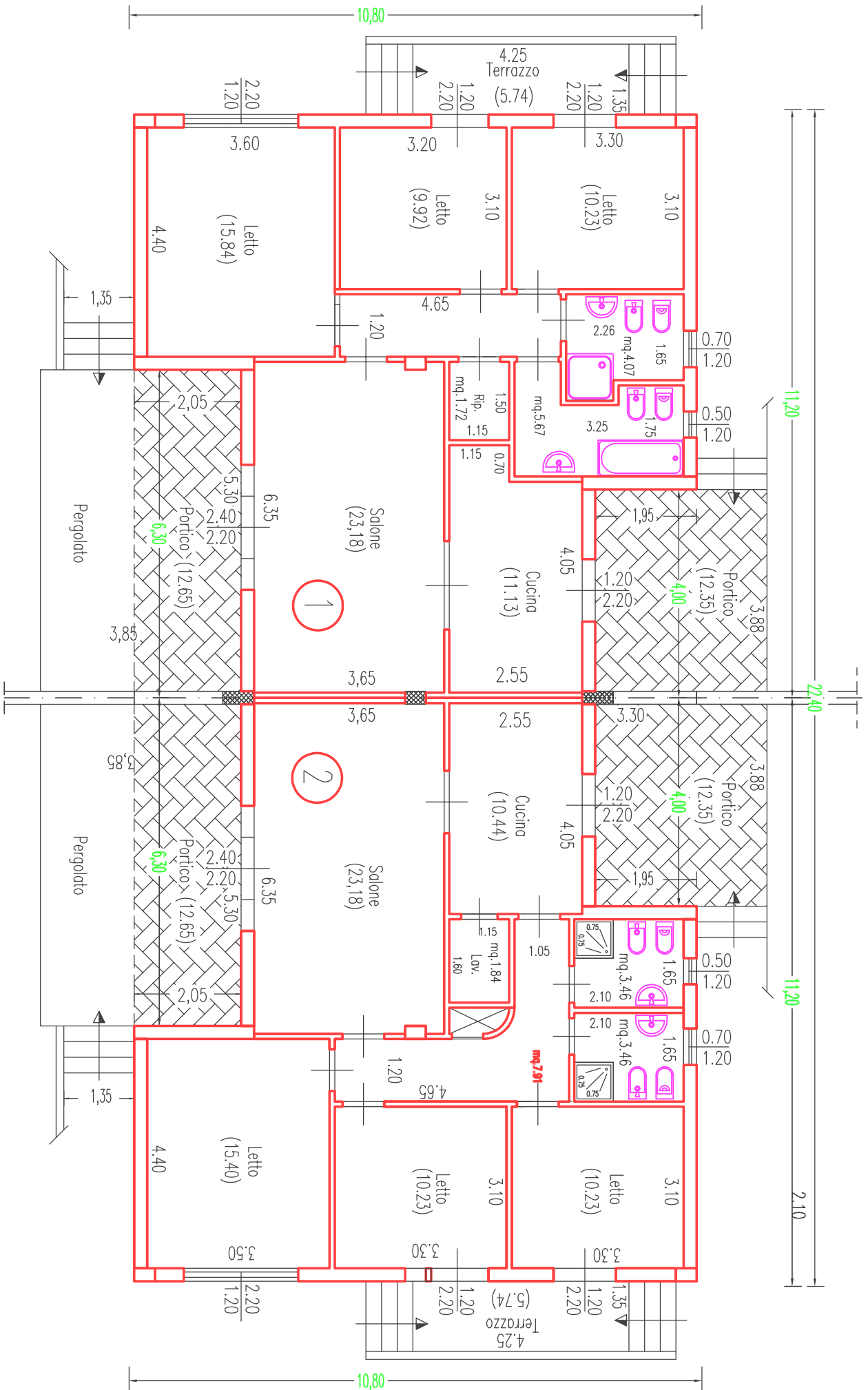
PIANTA DEL PIANO TERRA (Scala 1:100) tipologia per Villa "B" lotti da 2 a 6 (S.C.=mq. 209,35 + 50 (Portico); S.U.=mq. 175,00)
